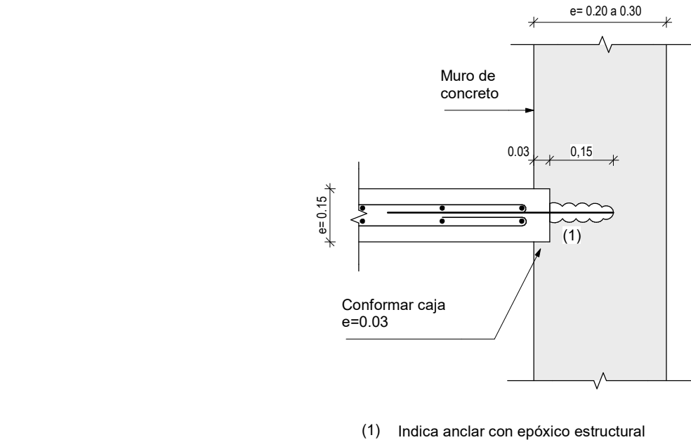
DETALLE 1 Escala 1 : 10
