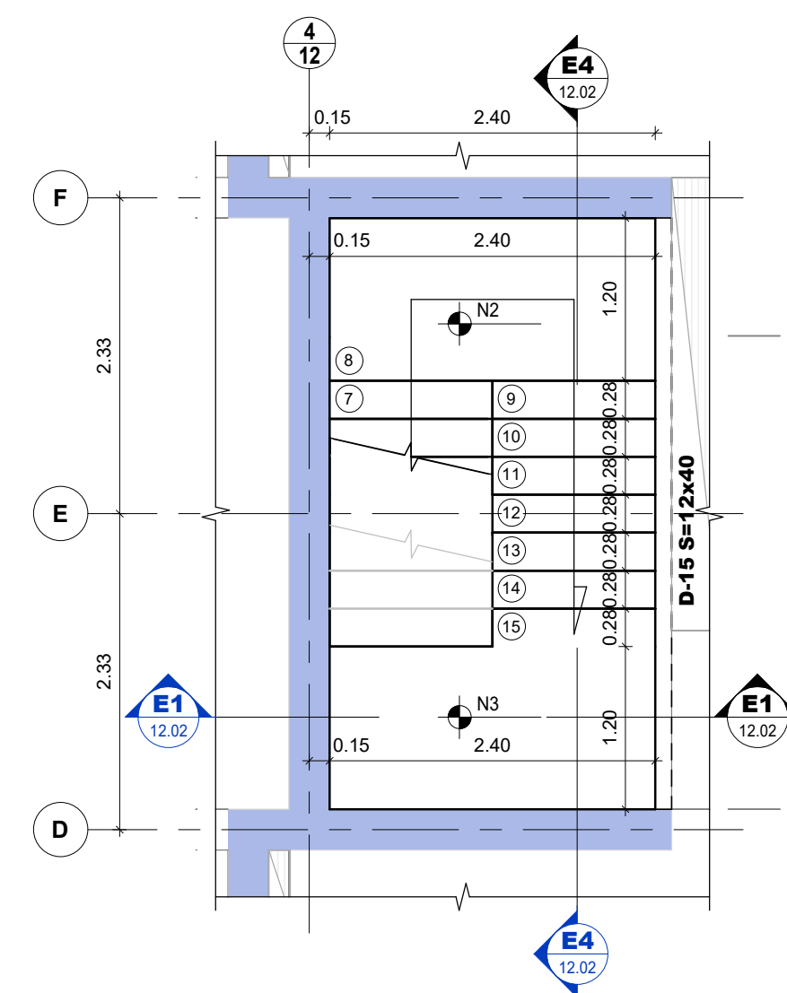
PLANTA LLEGADA ESCALERAS TIPO 1 Y 2 (PISO 3 A 28) Escala 1 : 50
