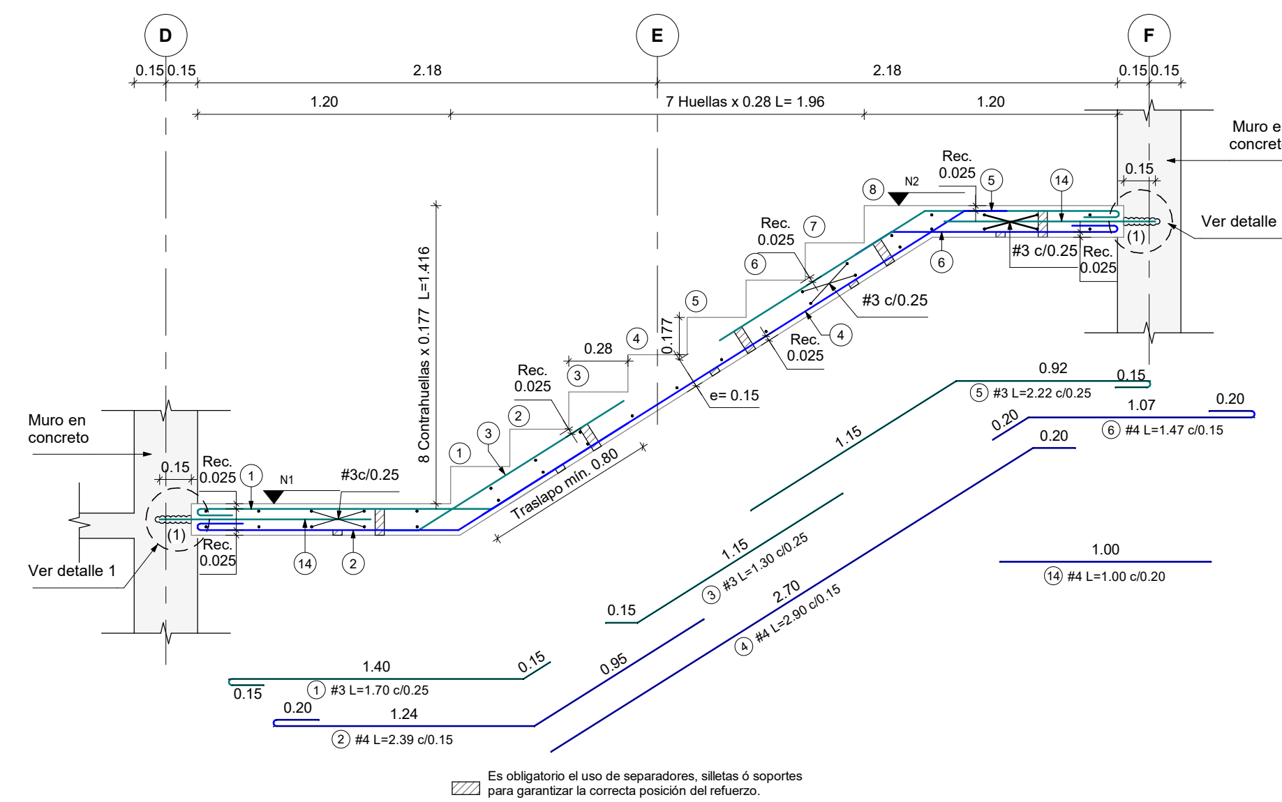
CORTE E-5 Escala 1 : 25
