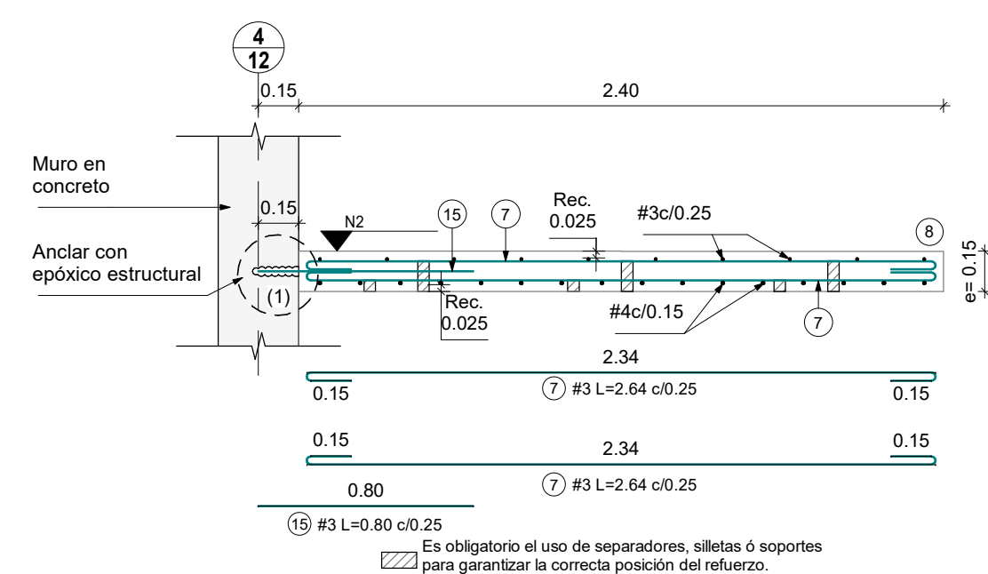
CORTE E-2 Escala 1 : 25
