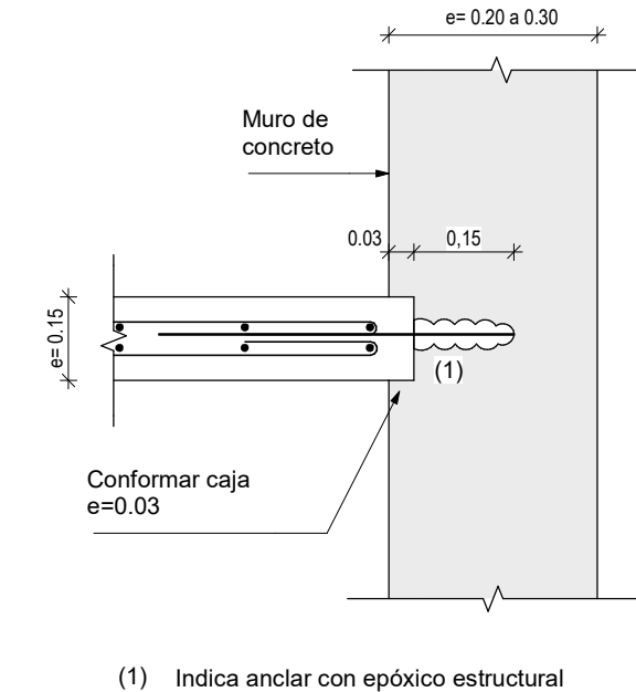
DETALLE 1 Escala 1 : 10
