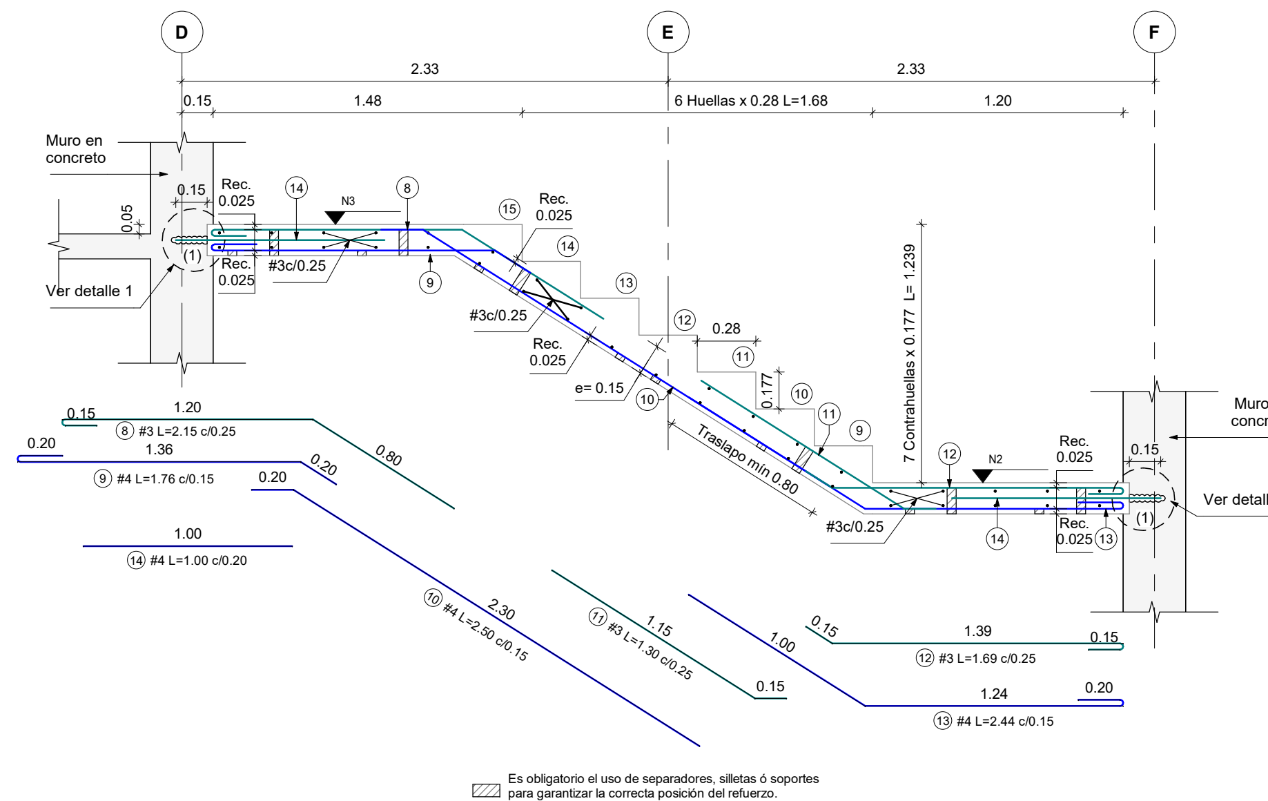
CORTE E-6 Escala 1 : 25
