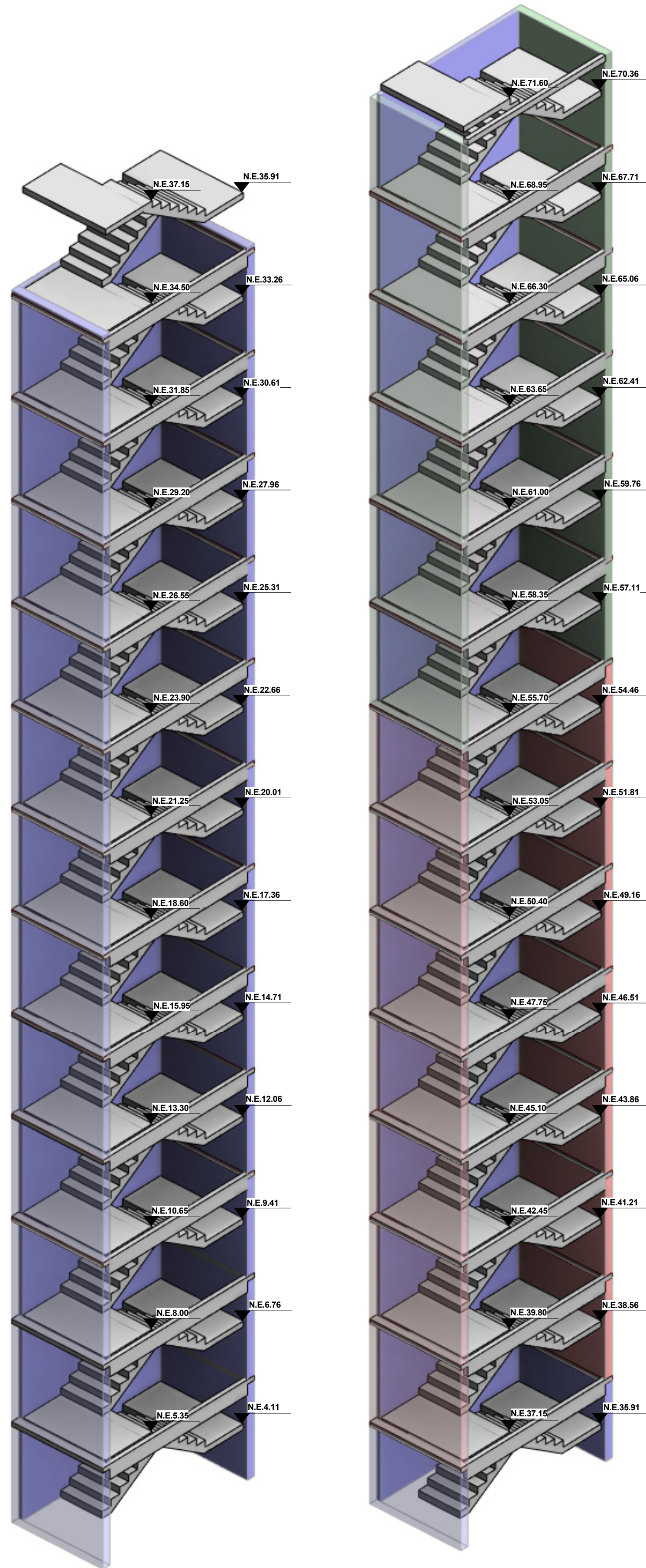
3D ESCALERAS TIPO 1 Y 2 DE PISO 2 A PISO 28 Sin escala
