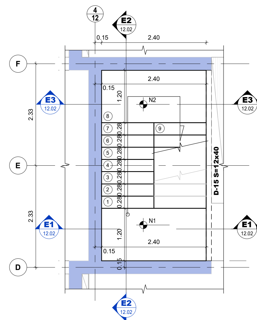
PLANTA ARRANQUE ESCALERAS TIPO 1 Y 2 (PISO 3 A 28) Escala 1 : 50
