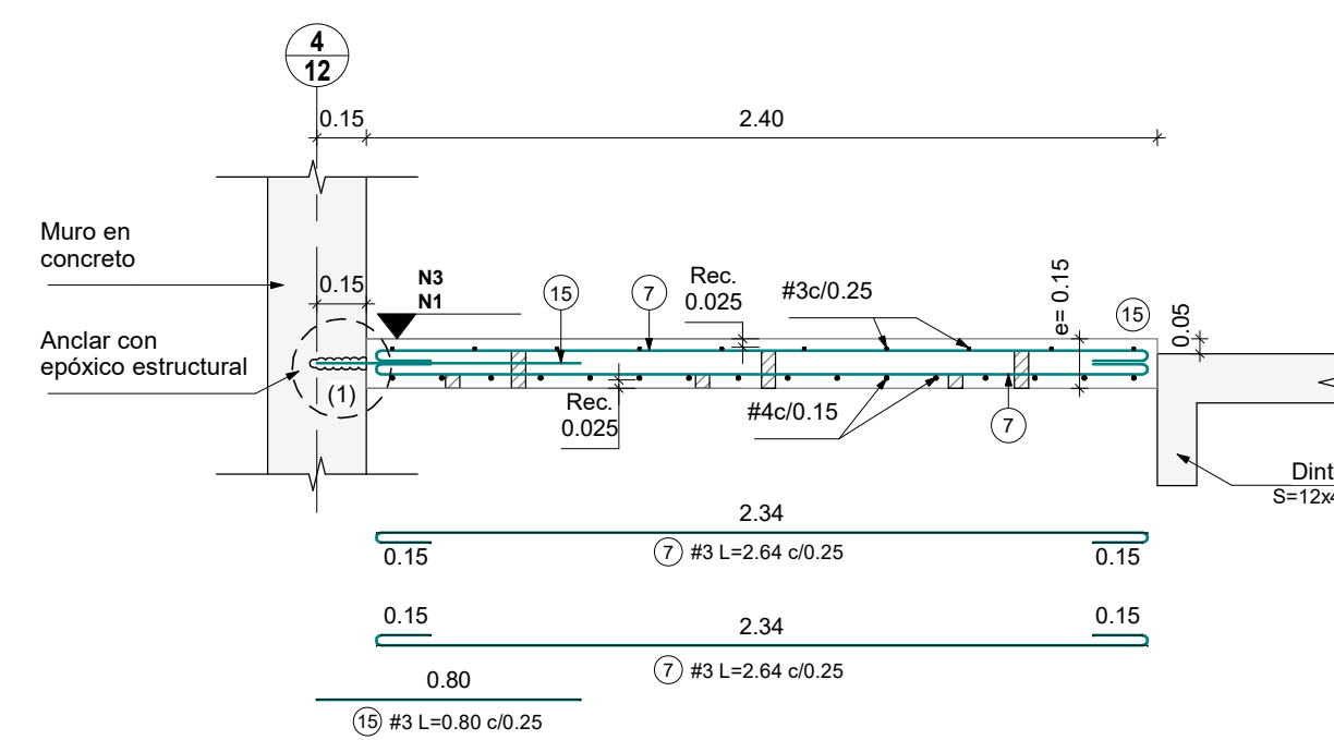
CORTE E-1 Escala 1 : 25
